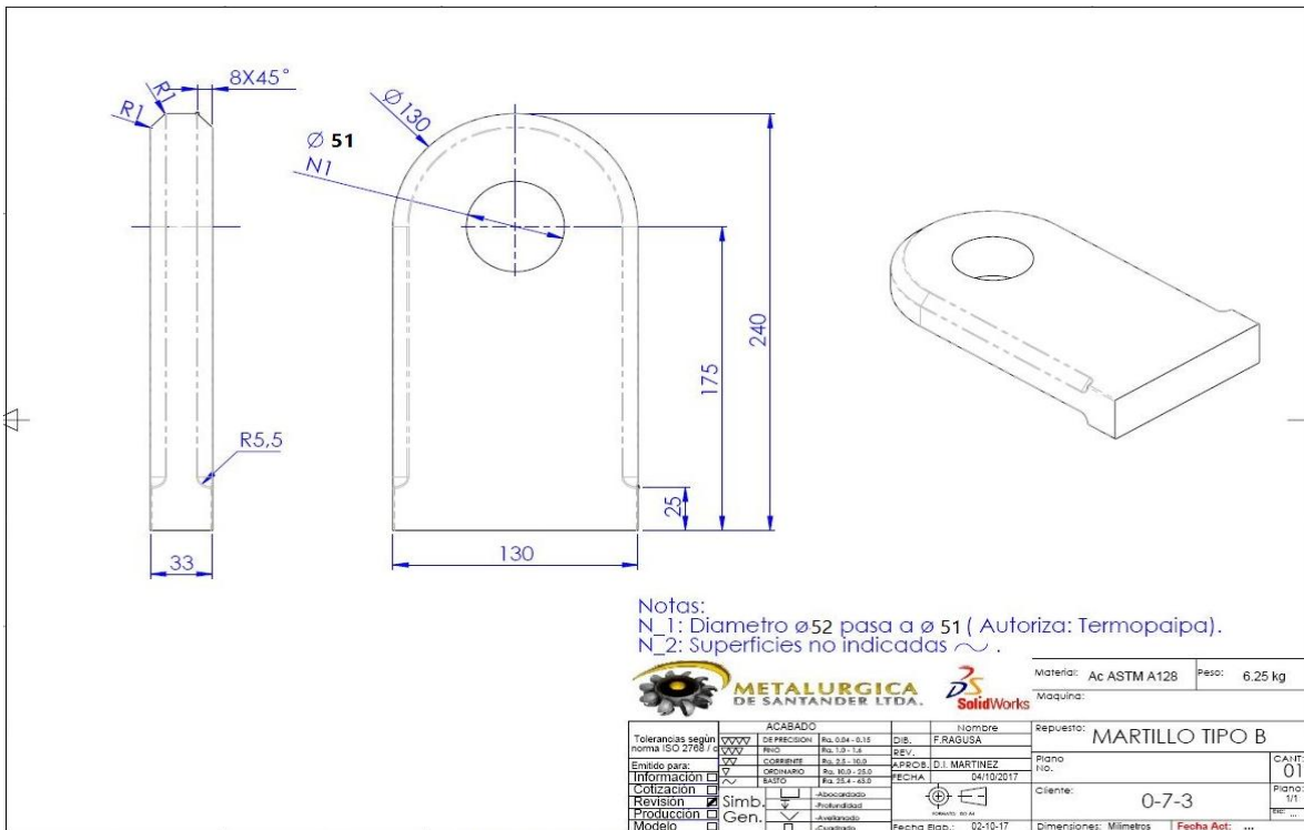
Plano martillo tipo B
