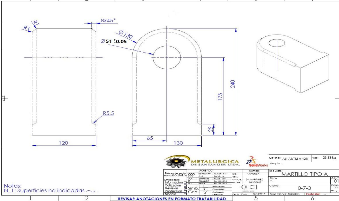
Plano martillo tipo A
