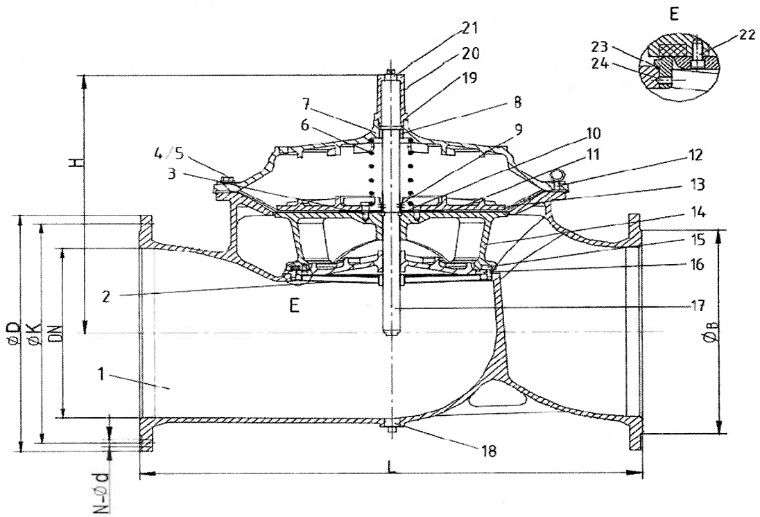
Detalle de la válvula anticipadora
