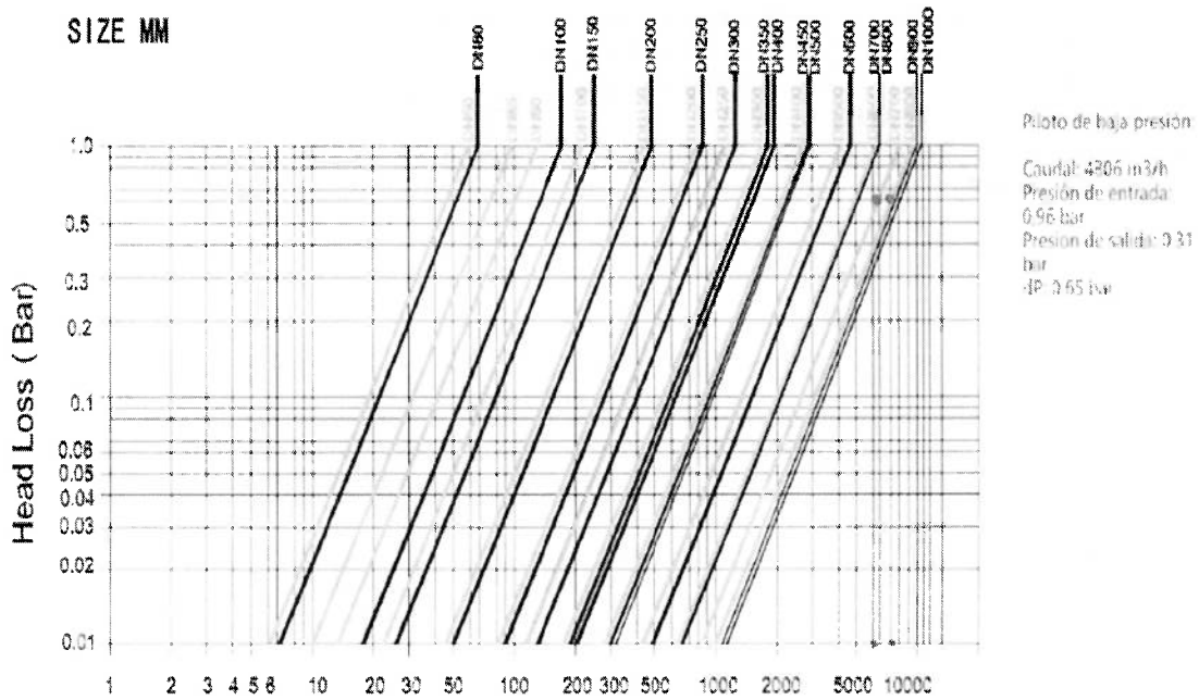
Curva de pérdida de presión vs Flujo válvula anticipadora. Correspondiente al la válvula DN700
