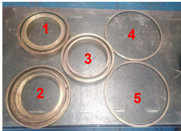
Imagen 6. Sellos en bronce a fabricar, lado libre
