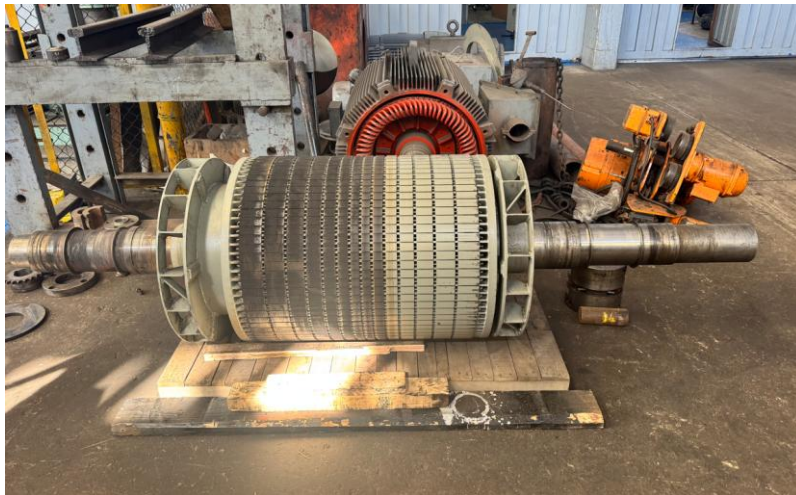
Imagen 3. Rotor
