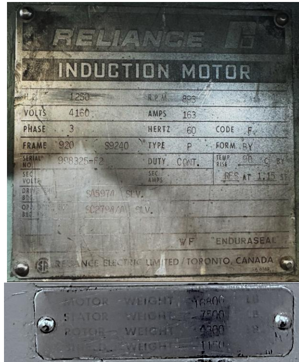
Imagen 1. Datos de placa y peso del motor
